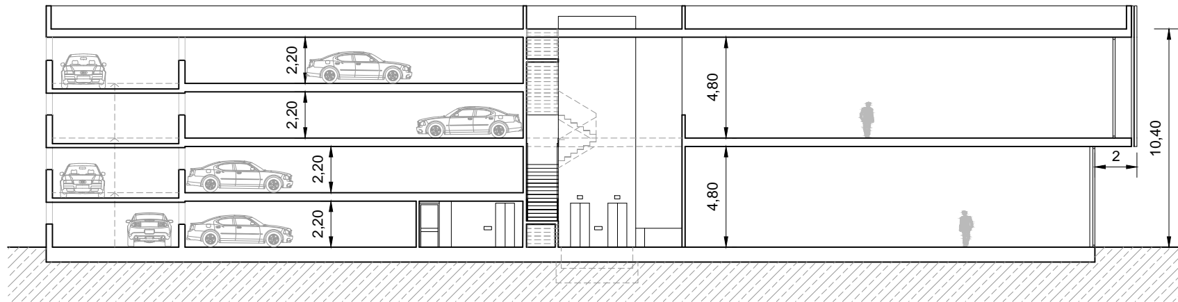
SECCIÓN TRANSVERSAL
